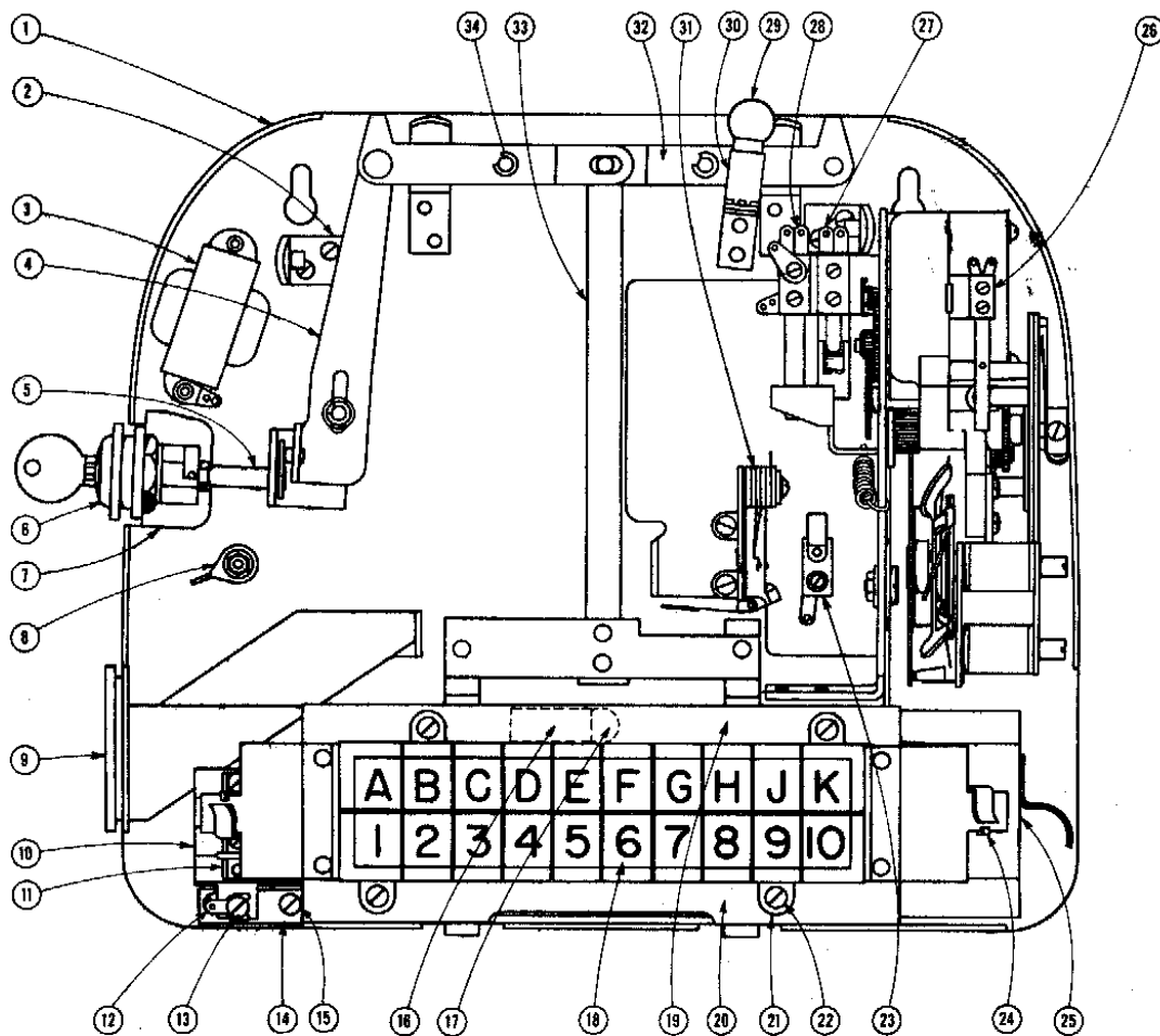
FIG. 21. BACK PLATE
